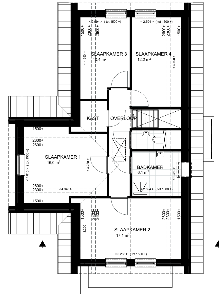
1e VERDIEPING
