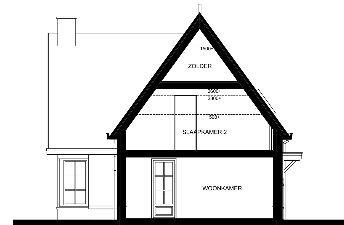
DOORSNEDE
