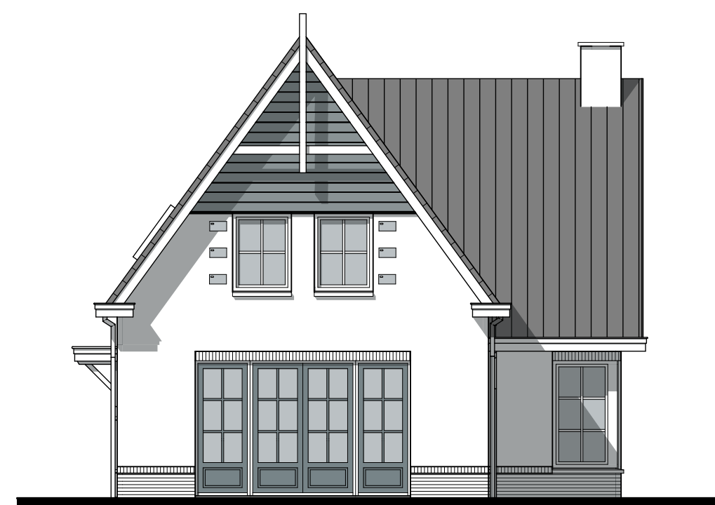
ACHTERGEVEL
