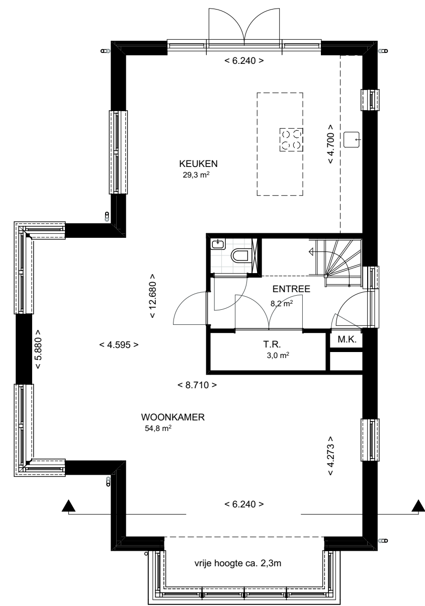
BEGANE GROND
