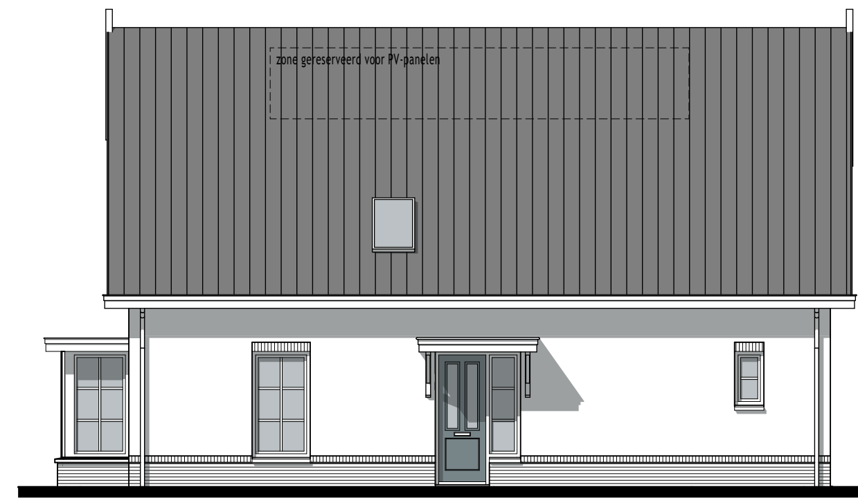
ZIJGEVEL RECHTS
