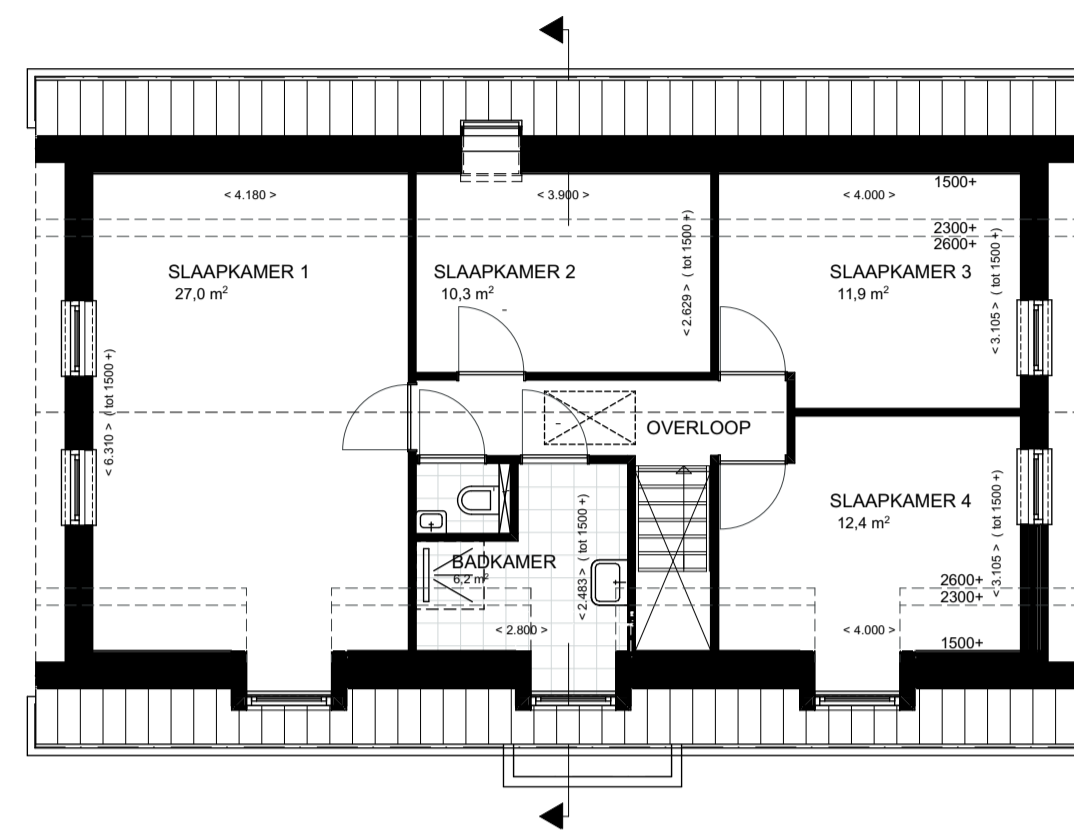
1e VERDIEPING
