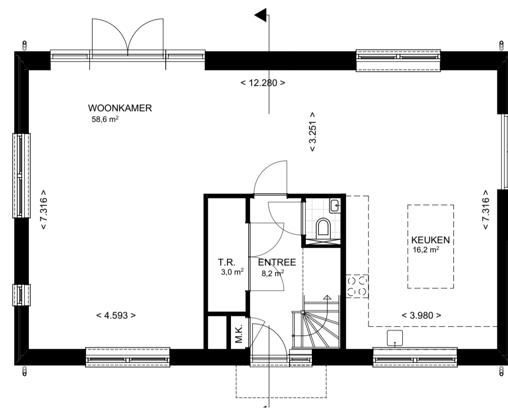
BEGANE GROND
