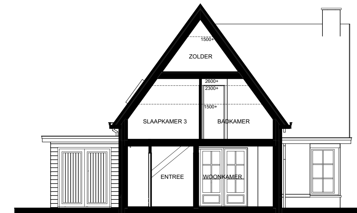
DOORSNEDE
