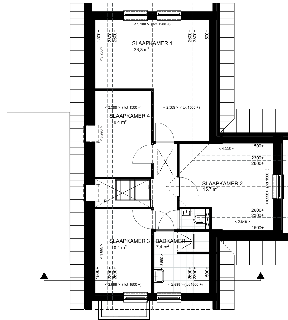
1e VERDIEPING
