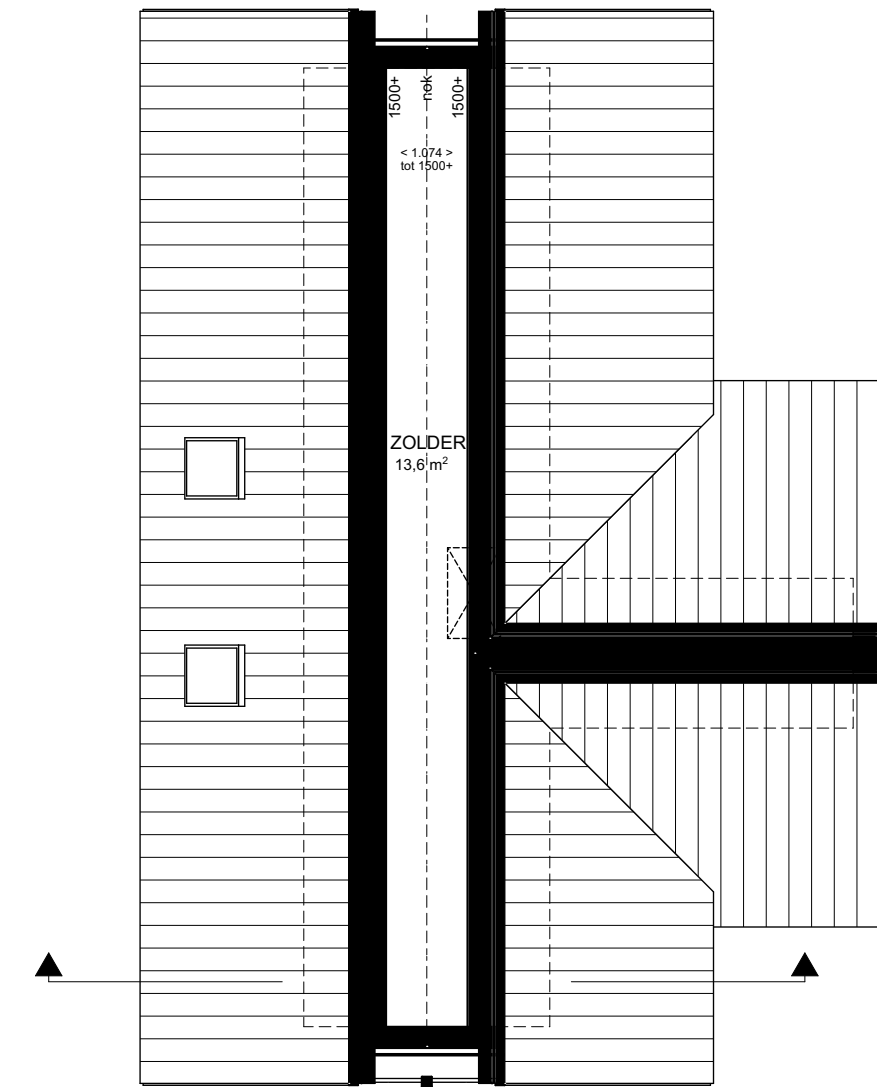
2e VERDIEPING
