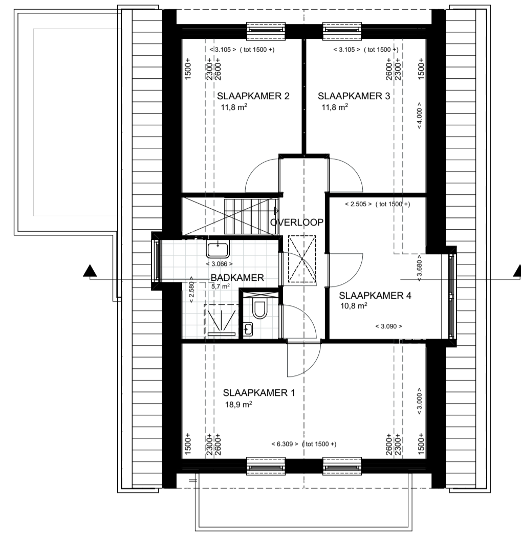
1e VERDIEPING
