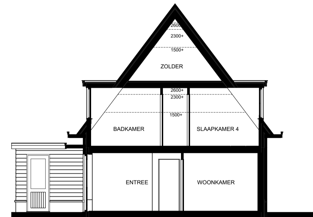
DOORSNEDE
