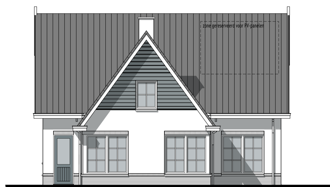
ZIJGEVEL RECHTS
