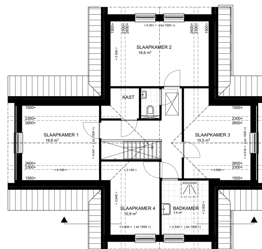
1e VERDIEPING
