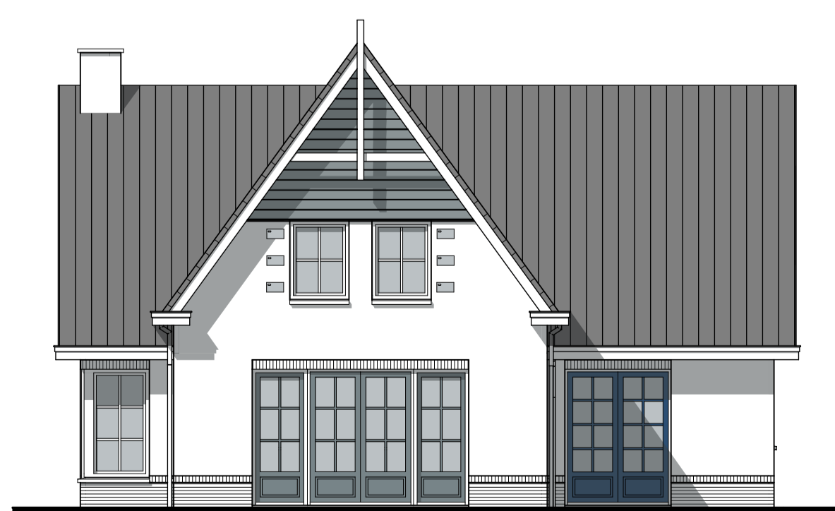
ACHTERGEVEL
